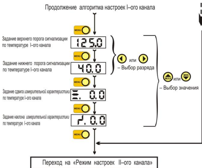
Рисунок 3 – Алгоритм режима настроек гигрометра IT-8-RHT (Общие настройки и настройки I-ого канала)
