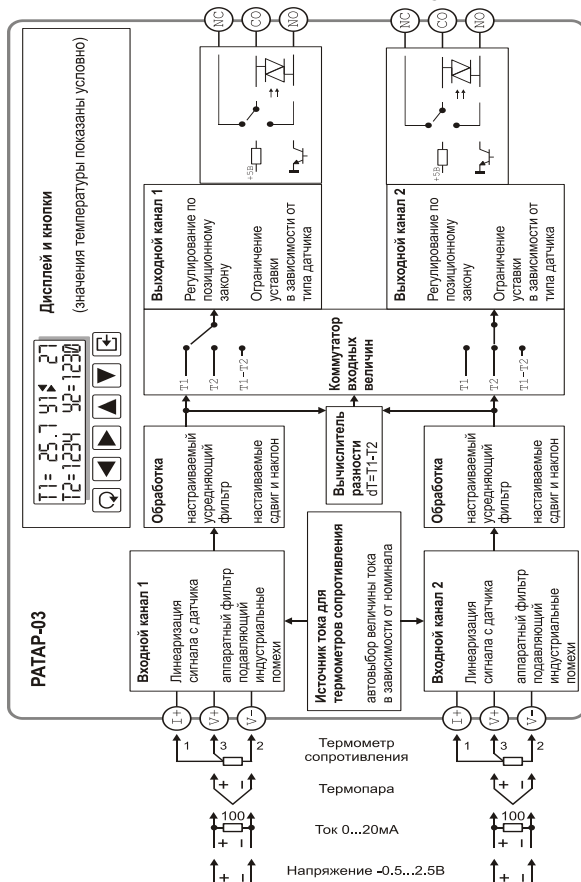
Рисунок 3 – Функциональная схема терморегулятора РАТАР-03.2УВ
