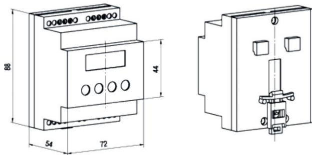
б) исполнение корпуса на DIN-рейку
