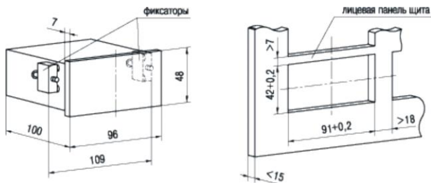
а) щитовое исполнение корпуса
